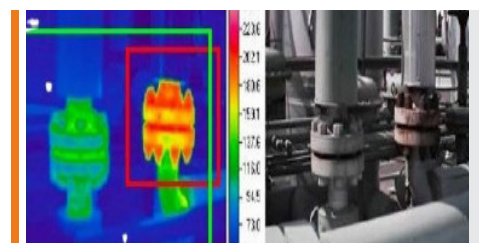
Thermal imaging
